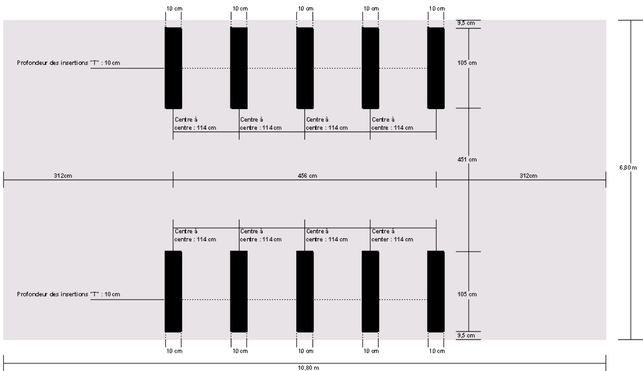
Schema 2 : Betonlaag of stabilisé
